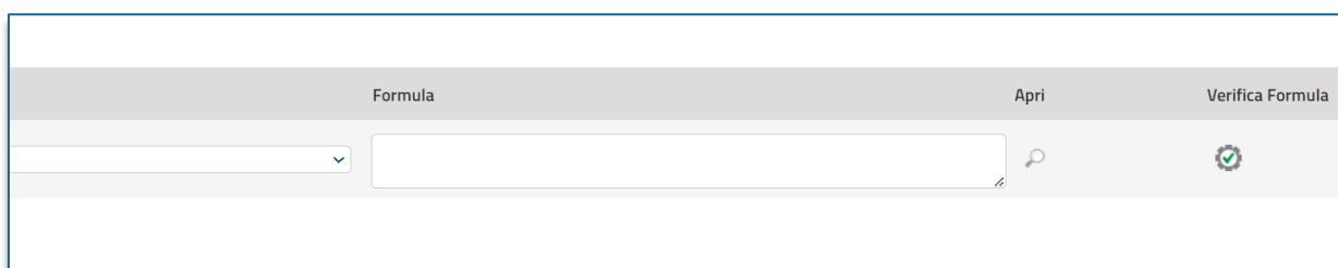
FIGURA 9 - DEFINIZIONE FORMULA
