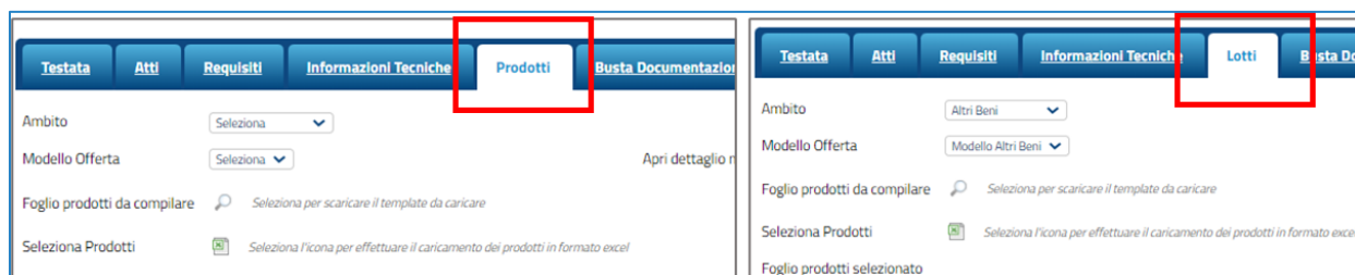
FIGURA 1 - PRODOTTI - LOTTI
