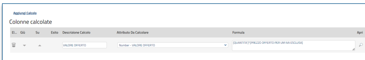
FIGURA 8 - COLONNE CALCOLATE
